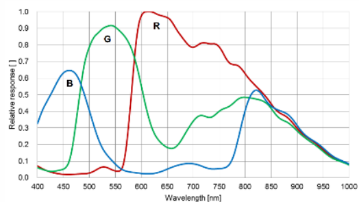
MV-CH089-10GC 量子效率
